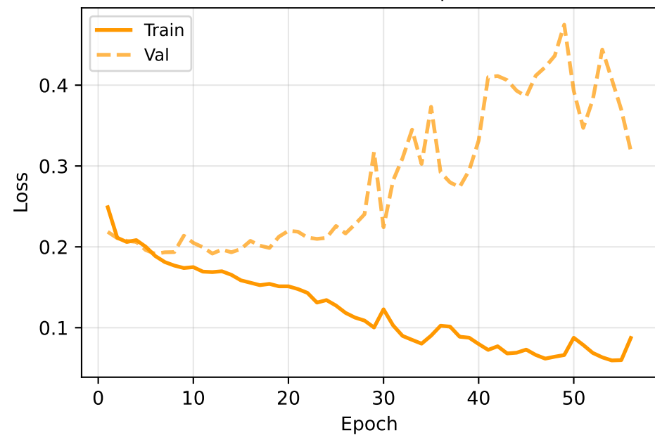
Total Loss ( \alpha \cdot \text{MSE} + \beta \cdot \text{BCE} )
